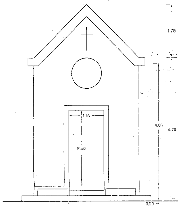
prospetto fronte
