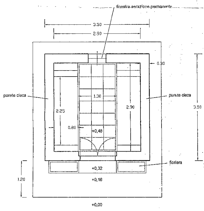
pianta tipo
