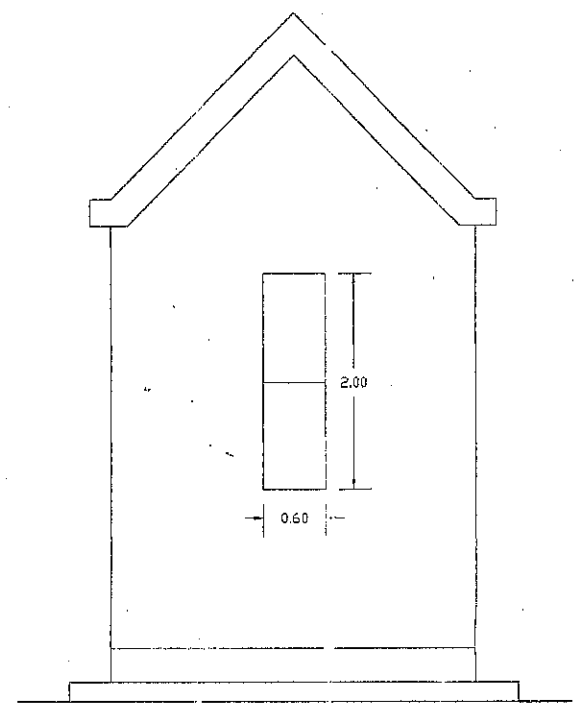
prospetto retro
